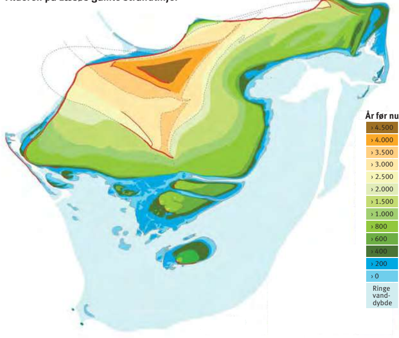
Alderen på Læsøs gamle strandlinjer
